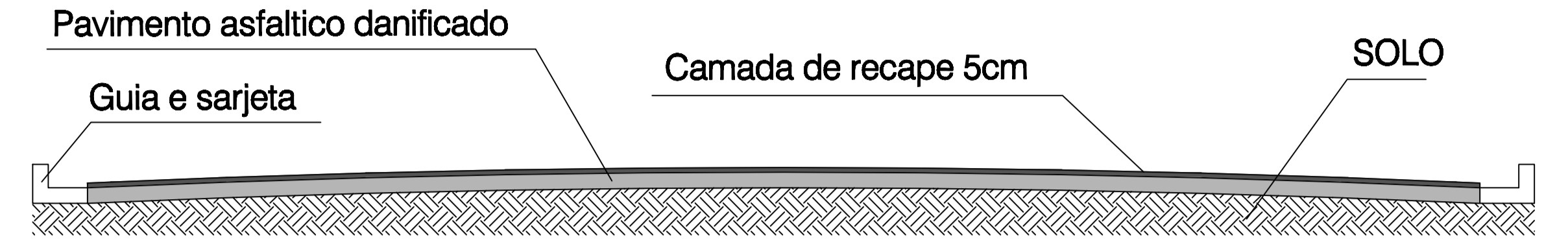
PERFIL DO RECAPE SEM ESCALA
