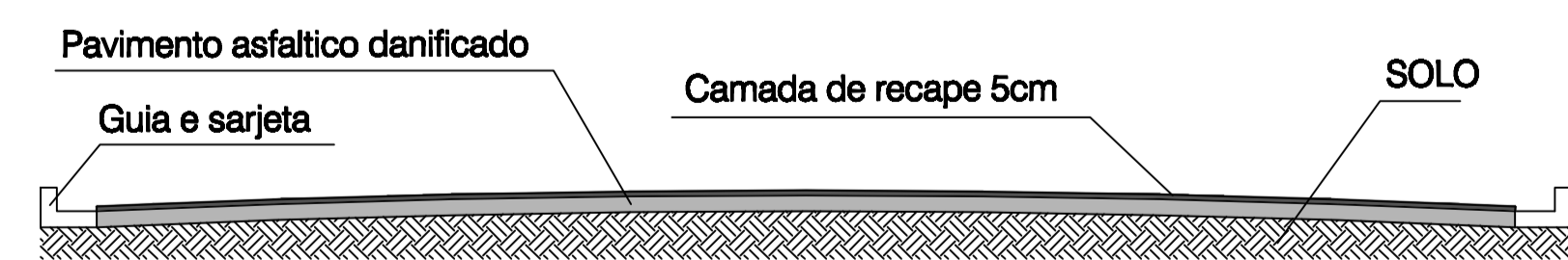
PERFIL DO RECAPE SEM ESCALA
